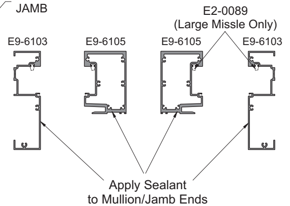
Detail 16 OXXO Frame
