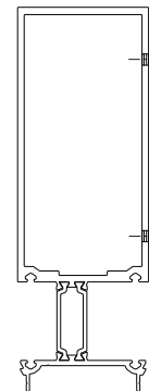
Jamb Mullion
