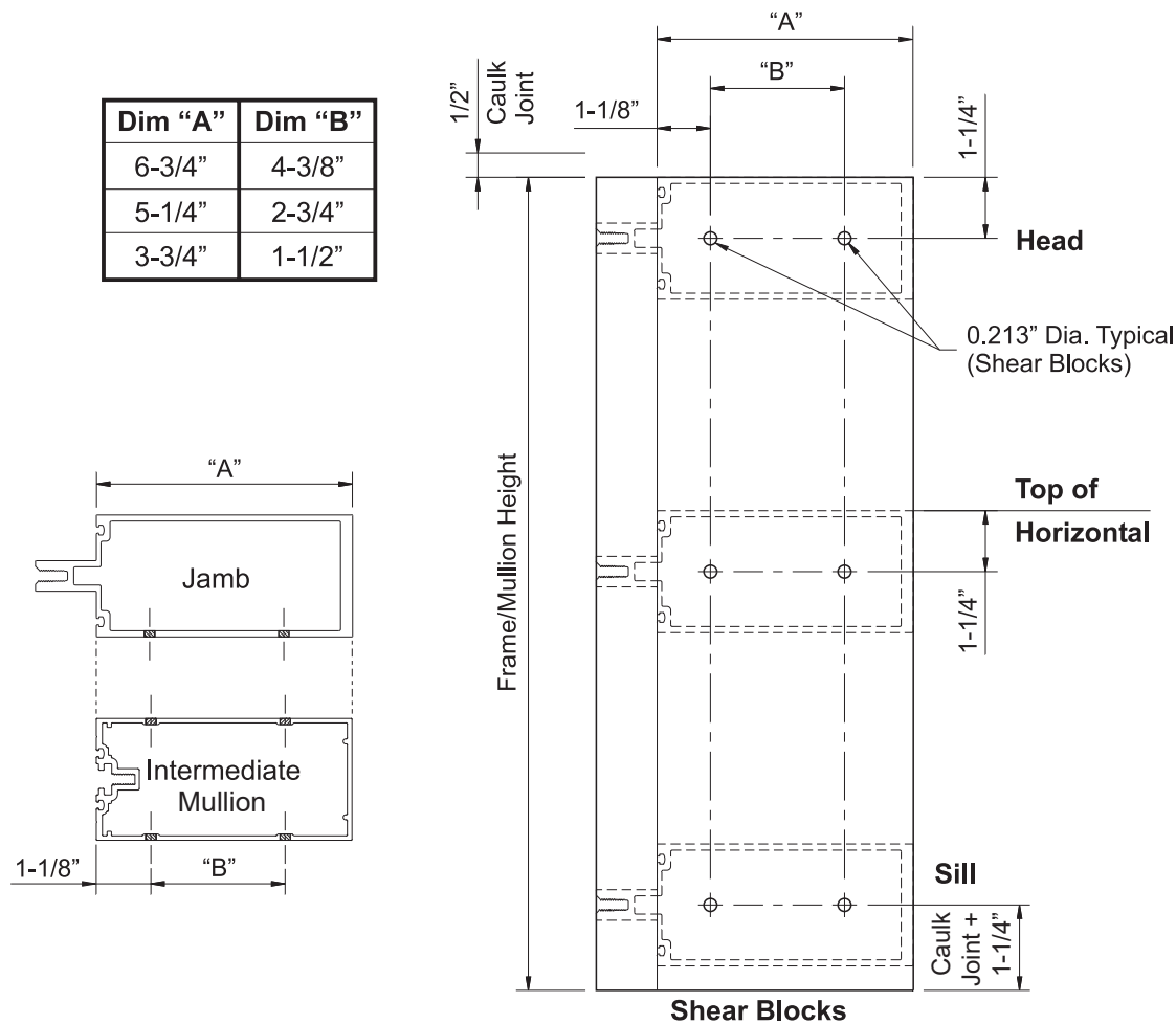
Detail 3 Door Jamb Mullion Fabrication
