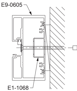
Jamb +70/-90 PSF*
