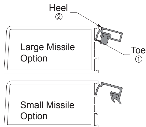
DETAIL 9a
