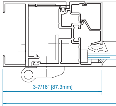
SECTION 9 Opp. w/ Optional Butt Hinge
