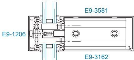
SECTION 2A OPEN BACK HORIZONTAL (1" Gl./1" Gl.)
