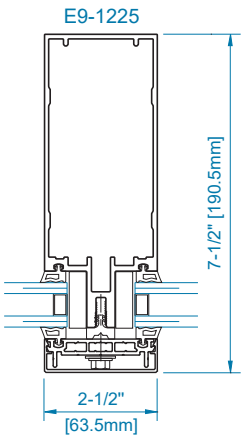
SECTION 6 VERTICAL (1" Gl.)
