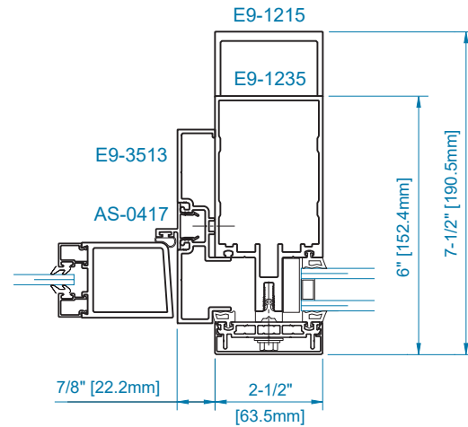
SECTION 9 DOOR JAMB
