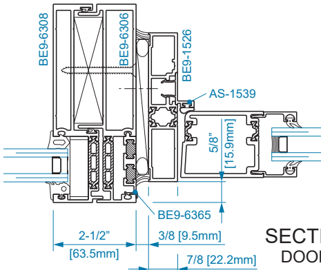
SECTION 21 DOOR JAMB @ TRANSOM
