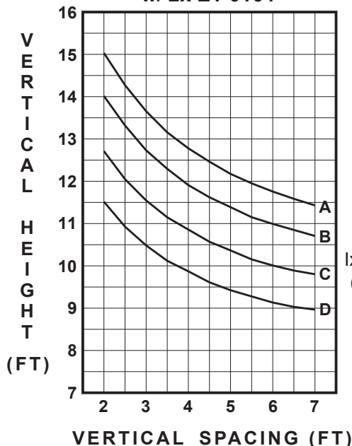
BE9-6303 / BE9-6306 w/ 2x E1-0164
