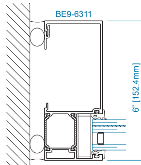
SECTION 59 O.G. JAMB
