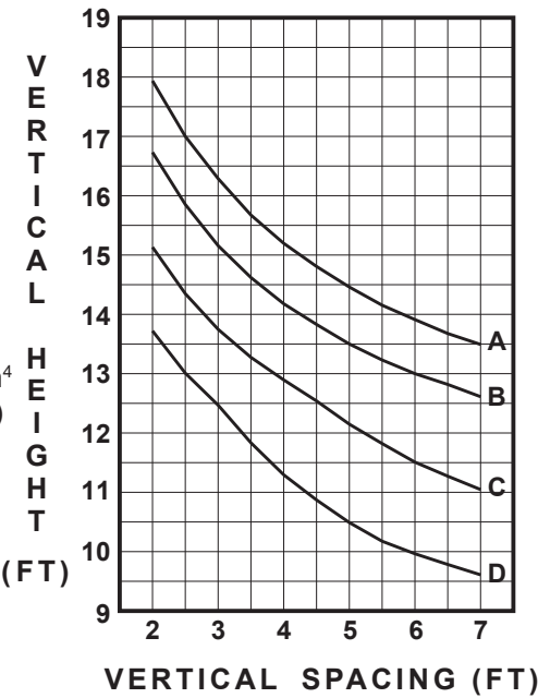
BE9-6360 / E9-6361 w/ E1-0164
