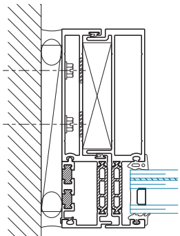
SECTION 71T DOOR JAMB @ TRANSOM
