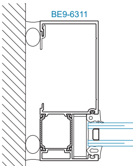
SECTION 9 O.G. JAMB
