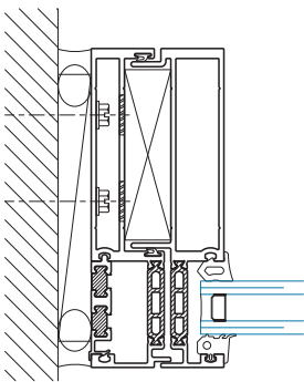
SECTION 21 DOOR JAMB @ TRANSOM
