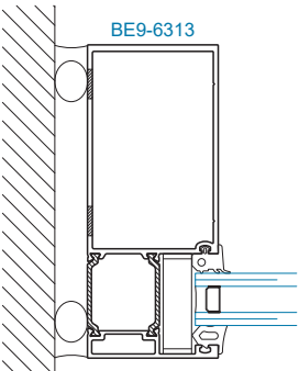
SECTION 9A TUBULAR O.G. JAMB
