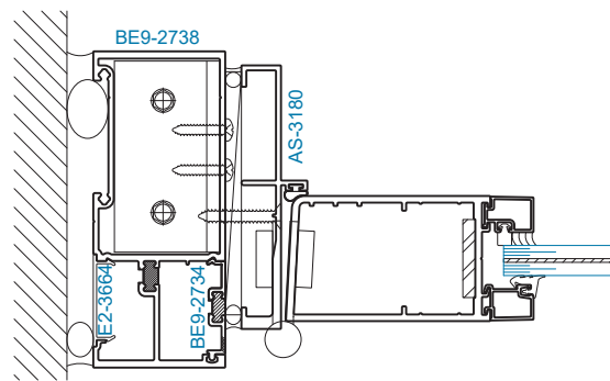
SECTION 14 DOOR JAMB w/o SIDELITE
