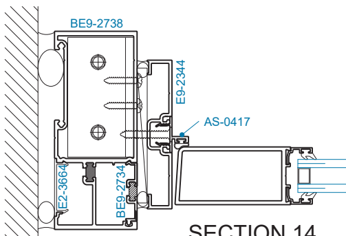
SECTION 14 DOOR JAMB w/o SIDELITE
