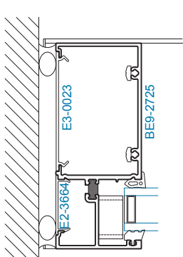
SECTION 4 JAMB
