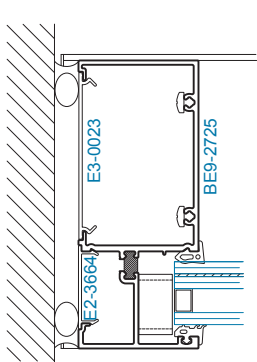
SECTION 4 JAMB
