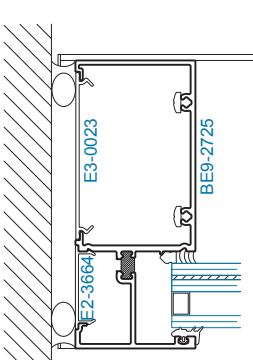
SECTION 4 JAMB
