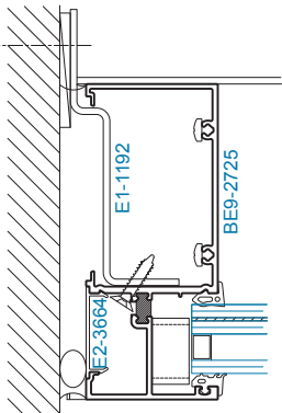
SECTION 4A JAMB
