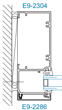
SECTION 5 JAMB
