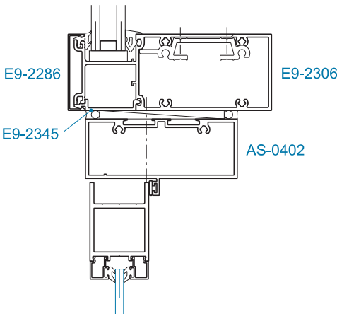
SECTION 15A TRANSOM BAR
