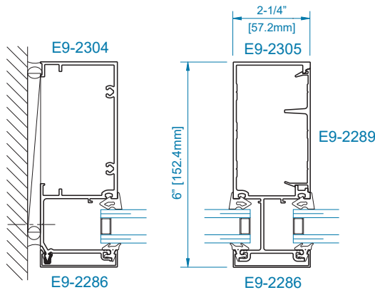
SECTION 5 JAMB
