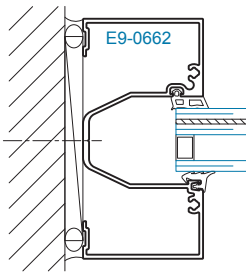
SECTION 4B JAMB +70/-90 PSF
