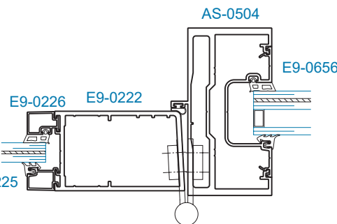
SECTION 13 DOOR JAMB w SIDELITE
