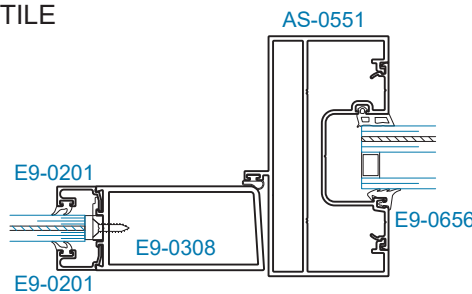
SECTION 13 DOOR JAMB w SIDELITE
