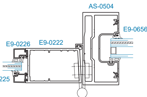
SECTION 13 DOOR JAMB w SIDELITE
