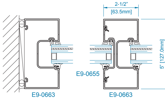
SECTION 4 JAMB ±50 PSF
