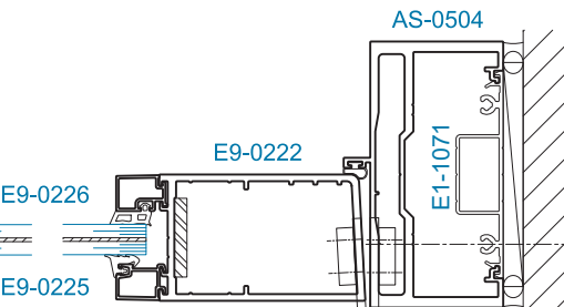
SECTION 10 JAMB w/o SIDELITE
