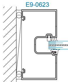
SECTION 4 JAMB ±50 PSF
