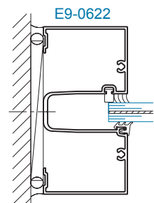
SECTION 4C JAMB (±70/-90 psf)
