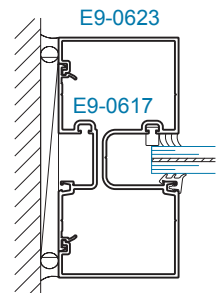
SECTION 4B JAMB (±70 psf)
