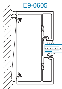
SECTION 4 JAMB (±70 psf)
