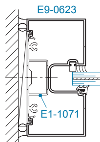
SECTION 4A JAMB (±70/-90 psf)
