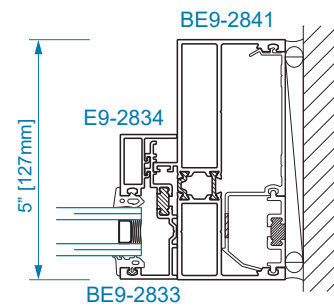
SECTION 32C DOOR JAMB AT TRANSOM
