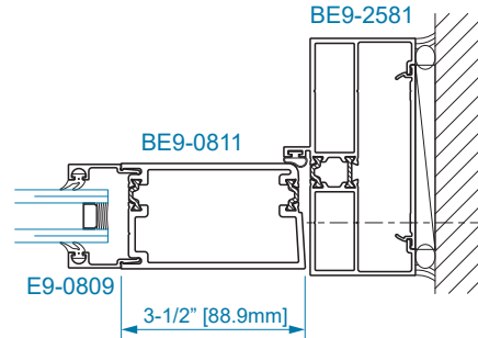
SECTION 23 HINGE JAMB
