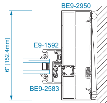
SECTION 32A DOOR JAMB AT TRANSOM
