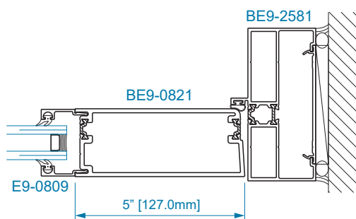
SECTION 28 LOCK JAMB
