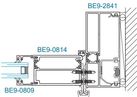
SECTION 33C HINGE JAMB
