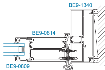
SECTION 33 HINGE JAMB
