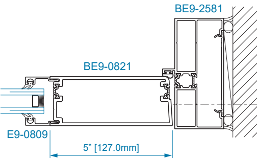
SECTION 28 HINGE JAMB
