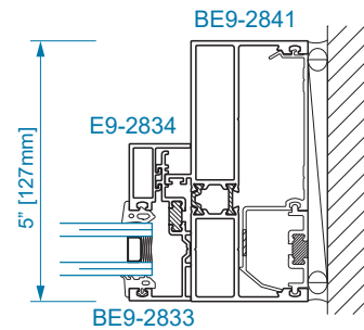
SECTION 32C DOOR JAMB AT TRANSOM
