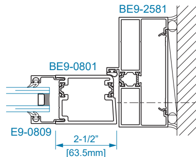
SECTION 15 LOCK JAMB
