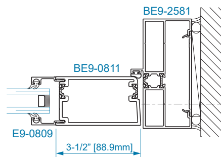
SECTION 23 LOCK JAMB
