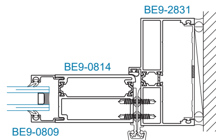
SECTION 33B HINGE JAMB
