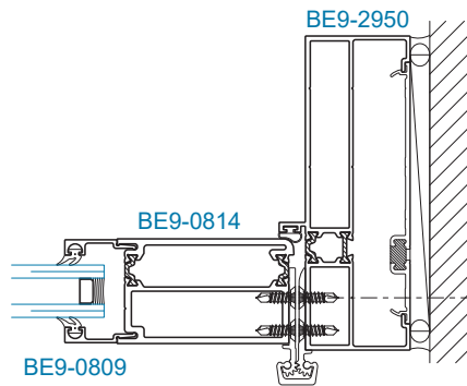
SECTION 33A HINGE JAMB
