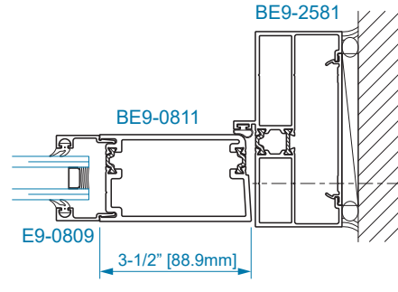
SECTION 23 HINGE JAMB
