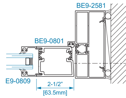
SECTION 15 HINGE JAMB
