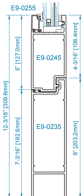
SECTION 2A OPTIONAL 12"
