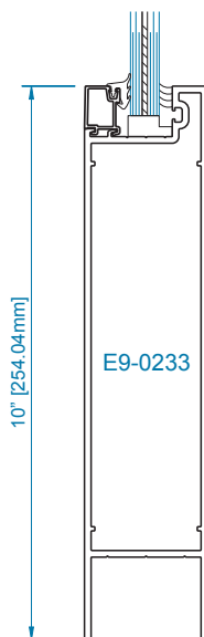
SECTION 3A OPTIONAL 10" BOTTOM RAIL*
