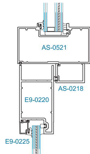
SECTION 4A OFFSET HUNG* (OHCC) 9/16" DOOR 1-5/16" TRANSOM
