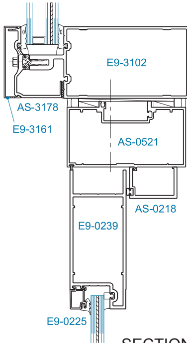
SECTION 3 YHC 300 OG W/ YHS 50 FI OFFSET HUNG (OHCC) 9/16" GLAZING
