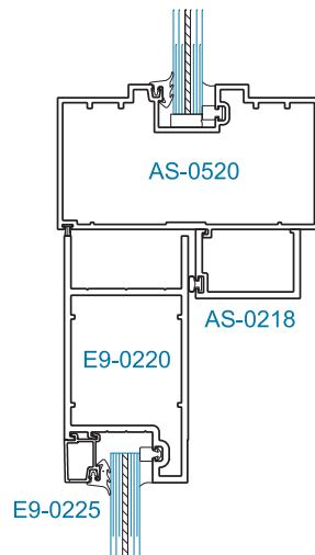
SECTION 4 OFFSET HUNG* (OHCC) 9/16" DOOR 9/16" TRANSOM
