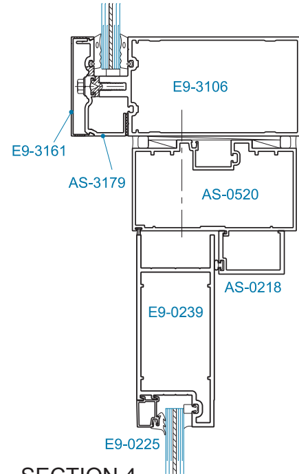
SECTION 4 YHC 300 OG W/ YHS 50 FS OFFSET HUNG (OHCC) 9/16" GLAZING
