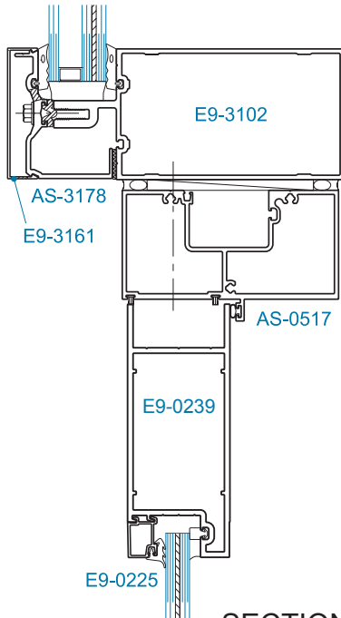
SECTION 1 YHC 300 OG W/ YHS 50 FI OFFSET HUNG 9/16" GLAZING
