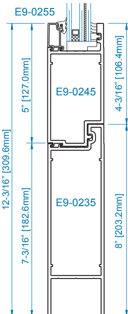
SECTION 2A OPTIONAL 12"
