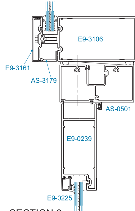
SECTION 2 YHC 300 OG W/ YHS 50 FS OFFSET HUNG 9/16" GLAZING
