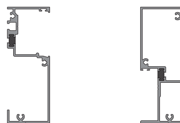
BE9-6203 Fixed Jamb
